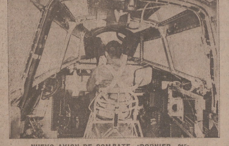
NUEVO AVION DE COMBATE «DORNIER 215» El avión de combate más moderno del arma aérea alemana es el «Dornier 215», que posee excelentes cualidades de vuelo
