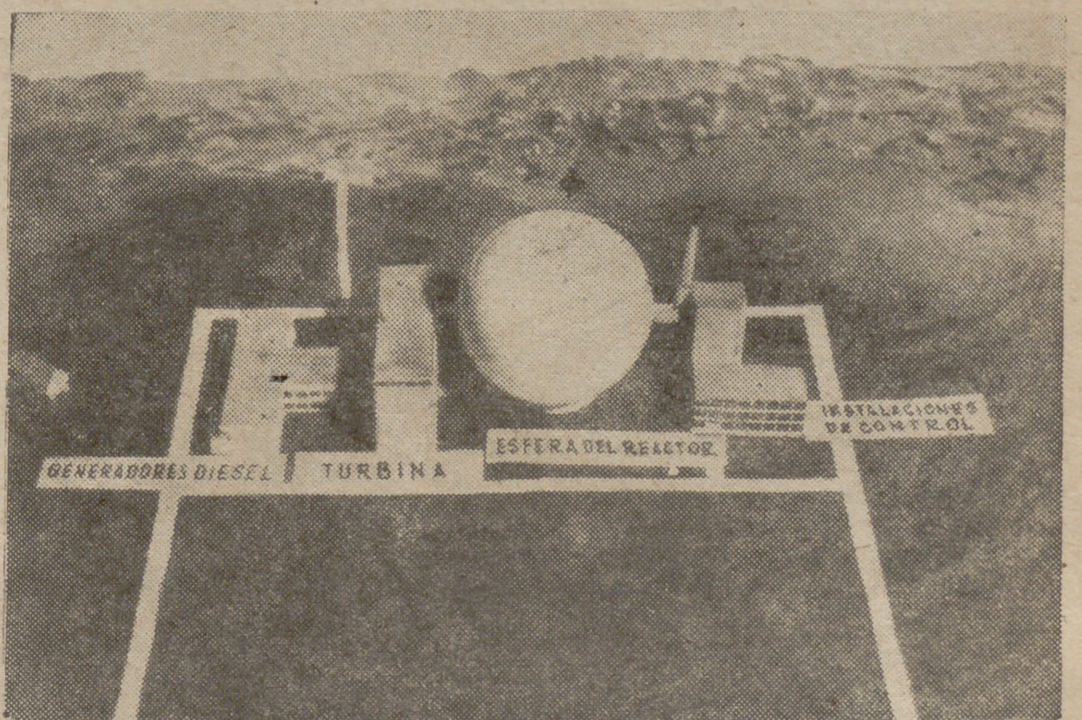
Esta es la maqueta de una nueva central de energía atómica, que será construida en Caithness (Escocia). Comprenderá un reactor capaz de desarrollar una gran energía calorífica y que convertirá el uranio ordinario en plutonio. La gran esfera central contendrá las sustancias radiactivas. Estas instalaciones suministrarán dentro de unos cinco años energía atómica para usos domésticos e industriales.
