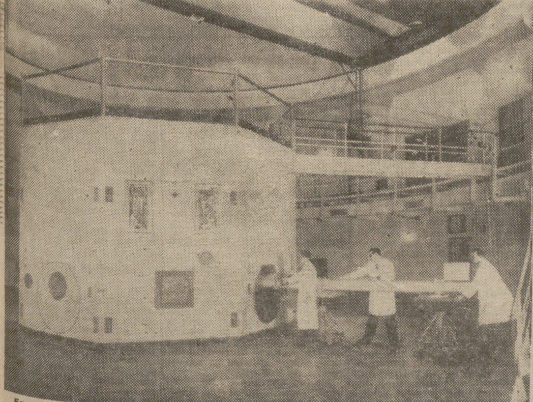
En el Laboratorio Nacional de Chicago ha sido instalado recientemente un nuevo reactor para investigaciones atómicas, que utiliza como "combustible" el uranio 235.
