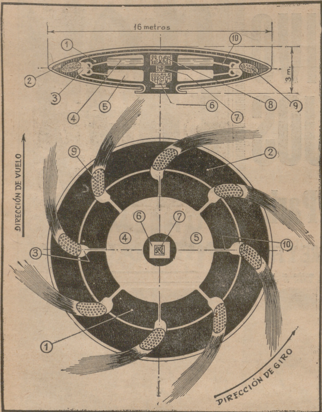
ESQUEMA DE UN PLATILLO VOLANTE.—1: Cuerpo móvil del "platillo".—2: Cuerpo giratorio del mismo.—3: Compresor con conducto de adhesión.—4: Depósito de alcohol.—5: Depósito de oxígeno.—6: Bloque de orientación y observación con televisión.—7: Cerebro electrónico con piloto automático.—8: Bloque de radar, dirección; emisor y receptor.—9: Desembocadura de turbo reactores.—10: Conductos de alimentación de alcohol y oxígeno.
