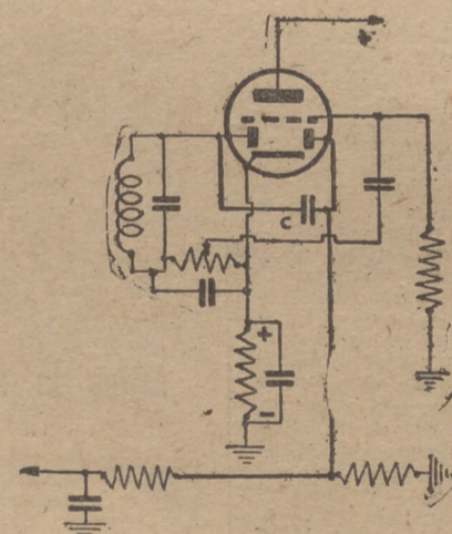
Fig. 136.—Esquema del control automático de sensibilidad retardado
