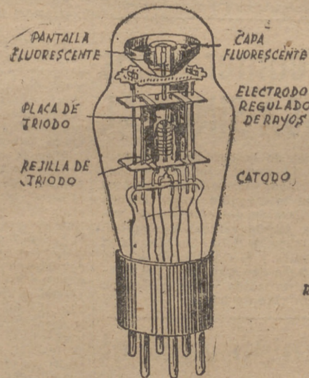
Fig. 137.—Lámpara "Ojo mágico"
