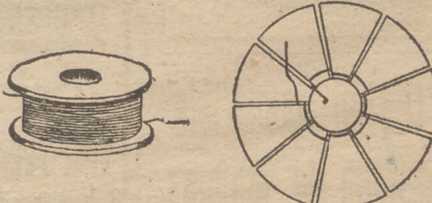
Fig. 6.—Bobina plana. Fig. 7.—Desarrollo de la bobina "fondo de cesta".
