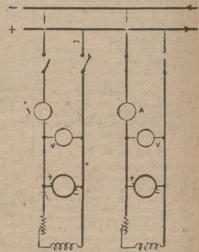
Esquema de acoplamiento de dinamos shunt
