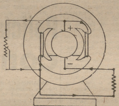
Esquema de dinamo compound
