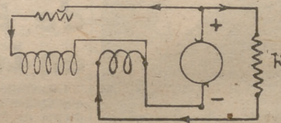
Esquema de dinamo compound
