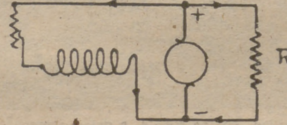
Esquema de dinamo derivación
