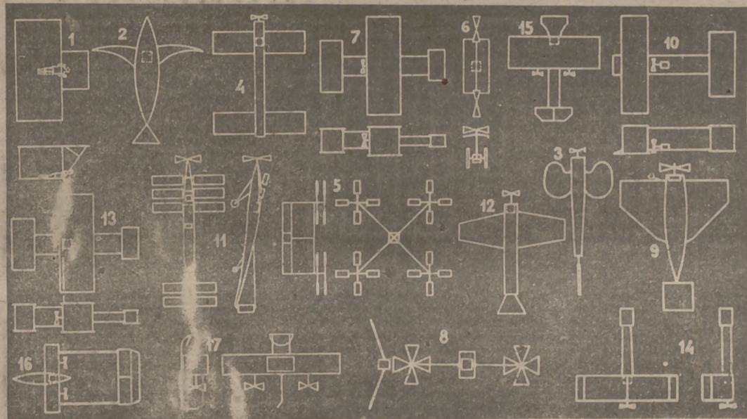
Esquemas de los principales tipos de aeroplanos y helicópteros: 1 y 17, Wright; 2, Bazin; 3 y 4, Bleriot; 5, Breguet; 6, Cornu; 7, De la Grange; 8, Duiaux; 9, Esnault-Pelterie; 10 y 11, Farman; 12, Gastambide-Mangin; 13, Kaplerer; 14, Santos-Dumont; 15, Seux; 16, De la Vaux.
