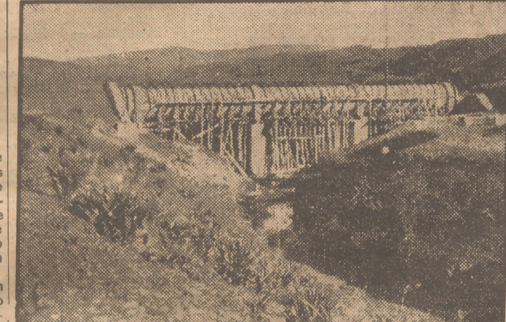
Sifón del Fresno, del trozo tercero del Canal del Viar.
