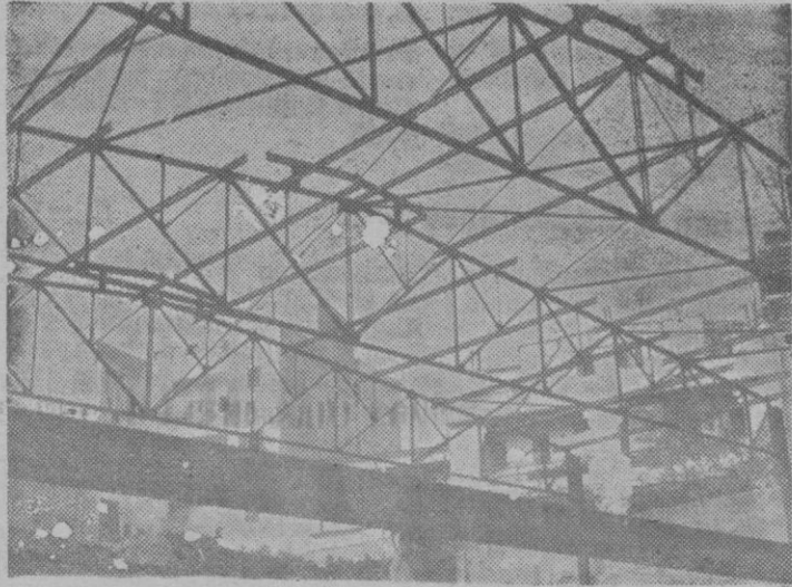
DETALLE DE PISO Y CUBIERTA PARA GARAJE. EN LA CALLE FRANCISCO SANCHO, DE PALMA.
