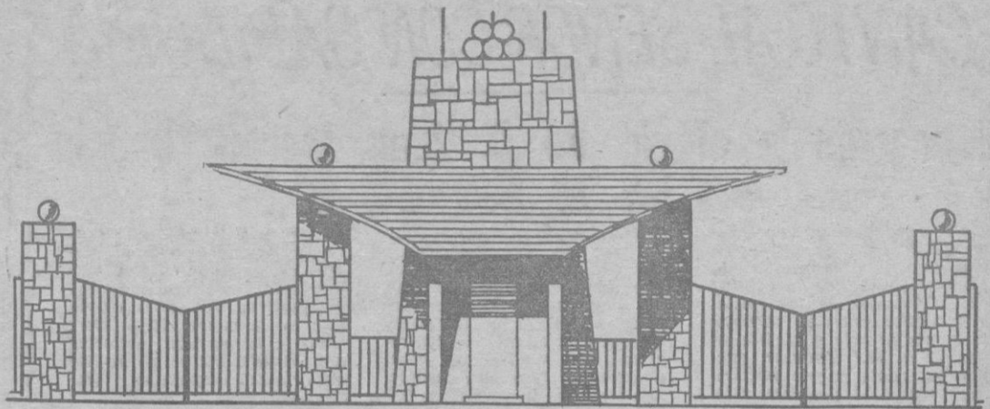
ALZADO POSTERIOR
