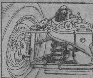
SUSPENSION DELANTERA A DOBLE EFECTO
