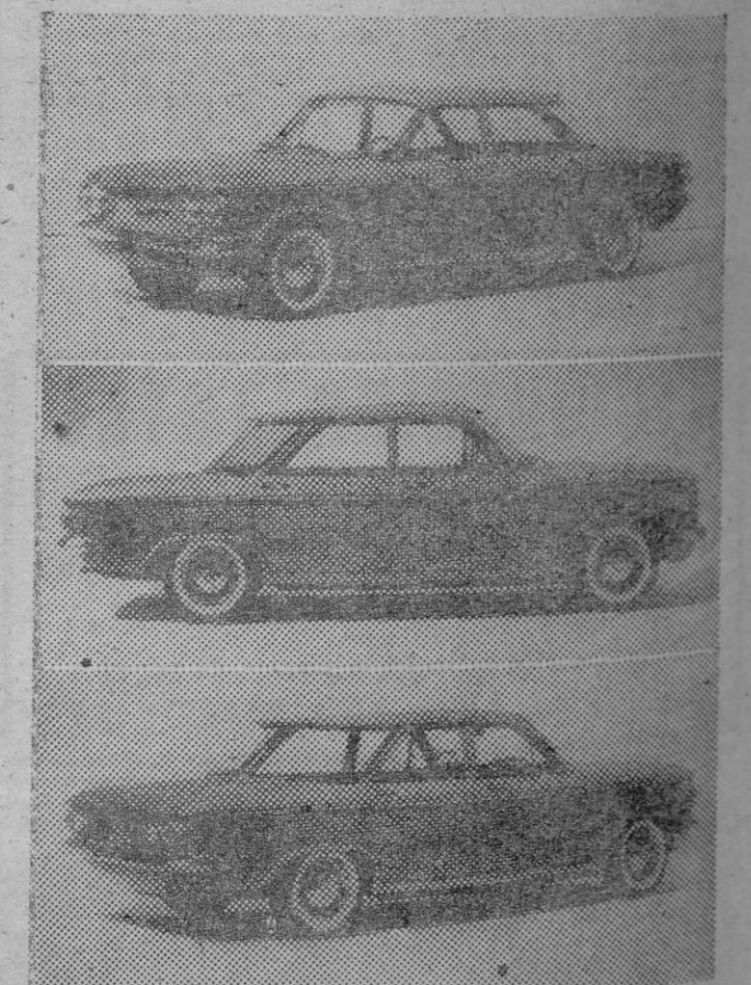
Respondiendo a los deseos de los americanos, que, según parece, están cansados de sus grandes coches, la casa Chevrolet ha ideado el pequeño coche solicitado, presentando en el Salón del Automóvil, de París, su automóvil «Compact». Este nuevo modelo tiene cuatro puertas, y está dotado con un motor de seis cilindros horizontales, con refrigeración por aire, con fuerza de 13 CV. Pesa 1.095 Kgs. y tiene una longitud de 1'57 metros por 1'70 de ancho. La casa constructora espera fabricar 300.000 unidades este año, de los 2 millones 165 mil vehículos que saldrán de sus fábricas.
