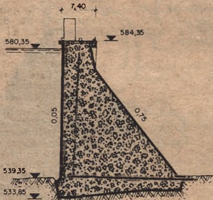
PRESA DE SANTOLEA
