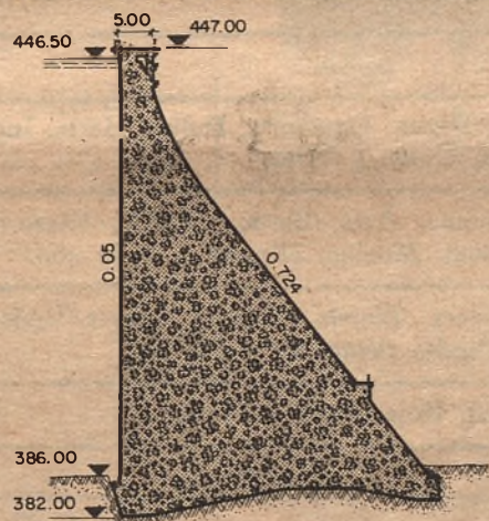
PRESA DE BARASONA
