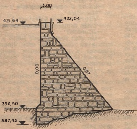
PRESA DE ARDISA
