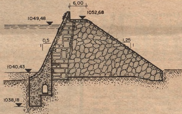
PRESA DE PLANDESCUN
