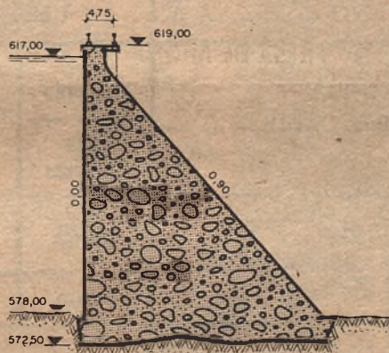
PRESA DE PENA
