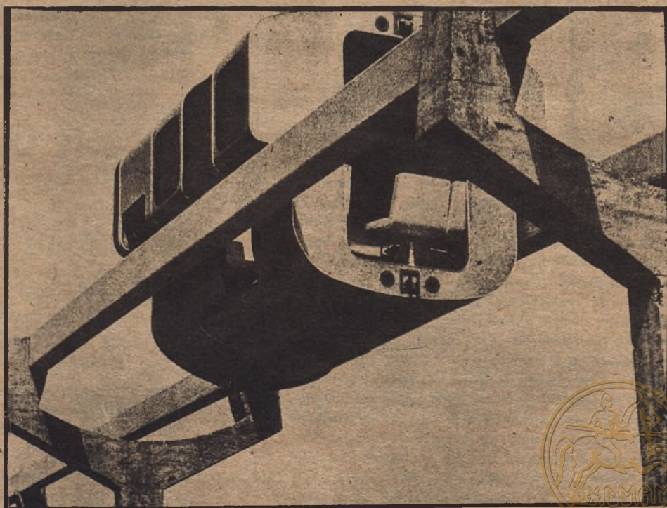
Desplazándose entre dos raíles a altas velocidades y con total seguridad, el "Aerotren" en un medio de transporte más eficaz que el tranvía o el autobús y apto, por lo menos, para desempeñar el mismo servicio que el "metro".
