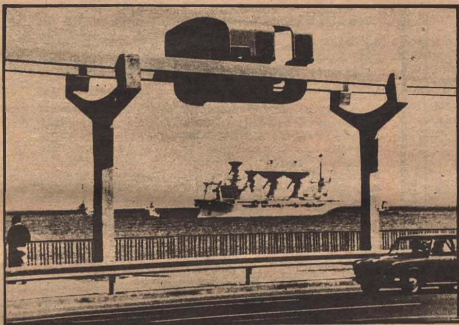
El "Aerotrán" circula a unos diez metros del suelo y los pilares de sustentación de los raíles ocupan poco espacio en su base. En la fotografía aparece el vagón utilizado para realizar las pruebas en Las Palmas de Gran Canaria, primera ciudad española que contará con este modernísimo sistema ideado por el inventor del "Talgo", don Alejandro Goicoechea.
