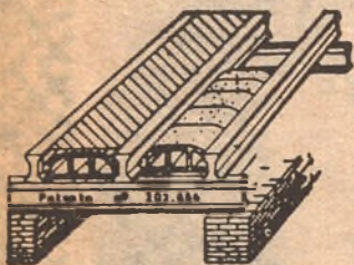
Vigueta especial Tipo 20 - A
