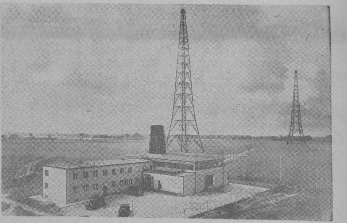
EDIFICIO Y ANTENAS DE LA POTENTE ESTACION DE LEIPZIG (ALEMANIA) 120 KW.
