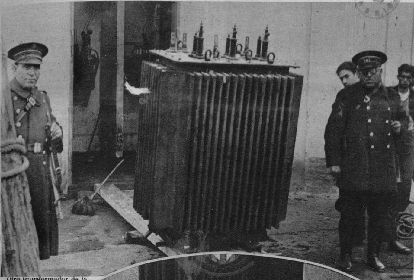
Otro transformador de la casa núm. 422 de la calle de Aragón, que sufrió desperfectos a causa de la explosión de una bomba
