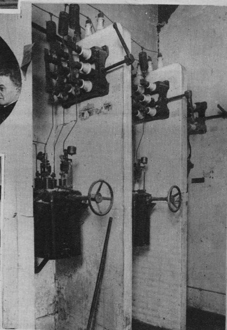
Las paredes del cuarto en que estaba colocado el transformador, quedaron cuarteadas, hundiéndose la techumbre. — (Fot. Merletti)
