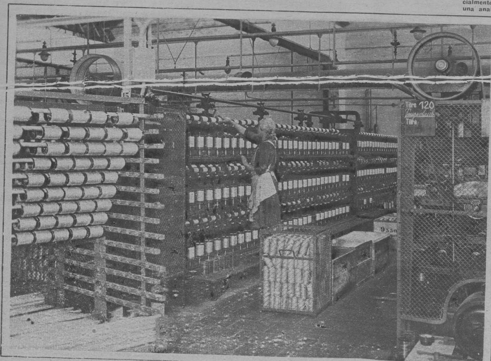
Máquinas para dar torsión a la seda artificial «Agfa Travis»
