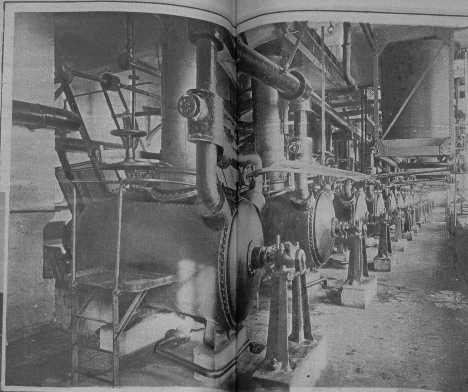
Calderas para la adición del xantogenato en una fábrica alemana de la «Agfa»
