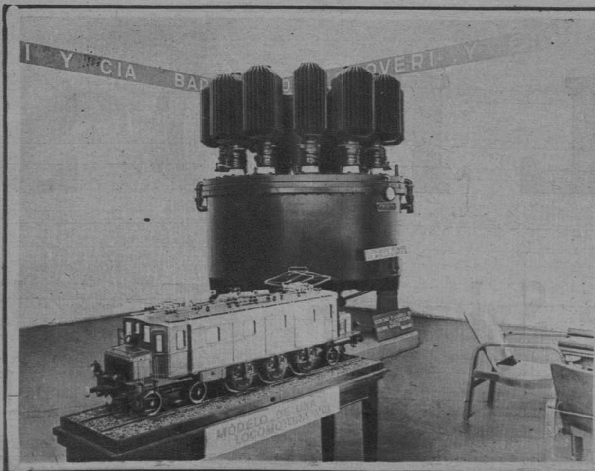
Rectificador de mercurio, tipo 6.400 A. y 1.500 V.
