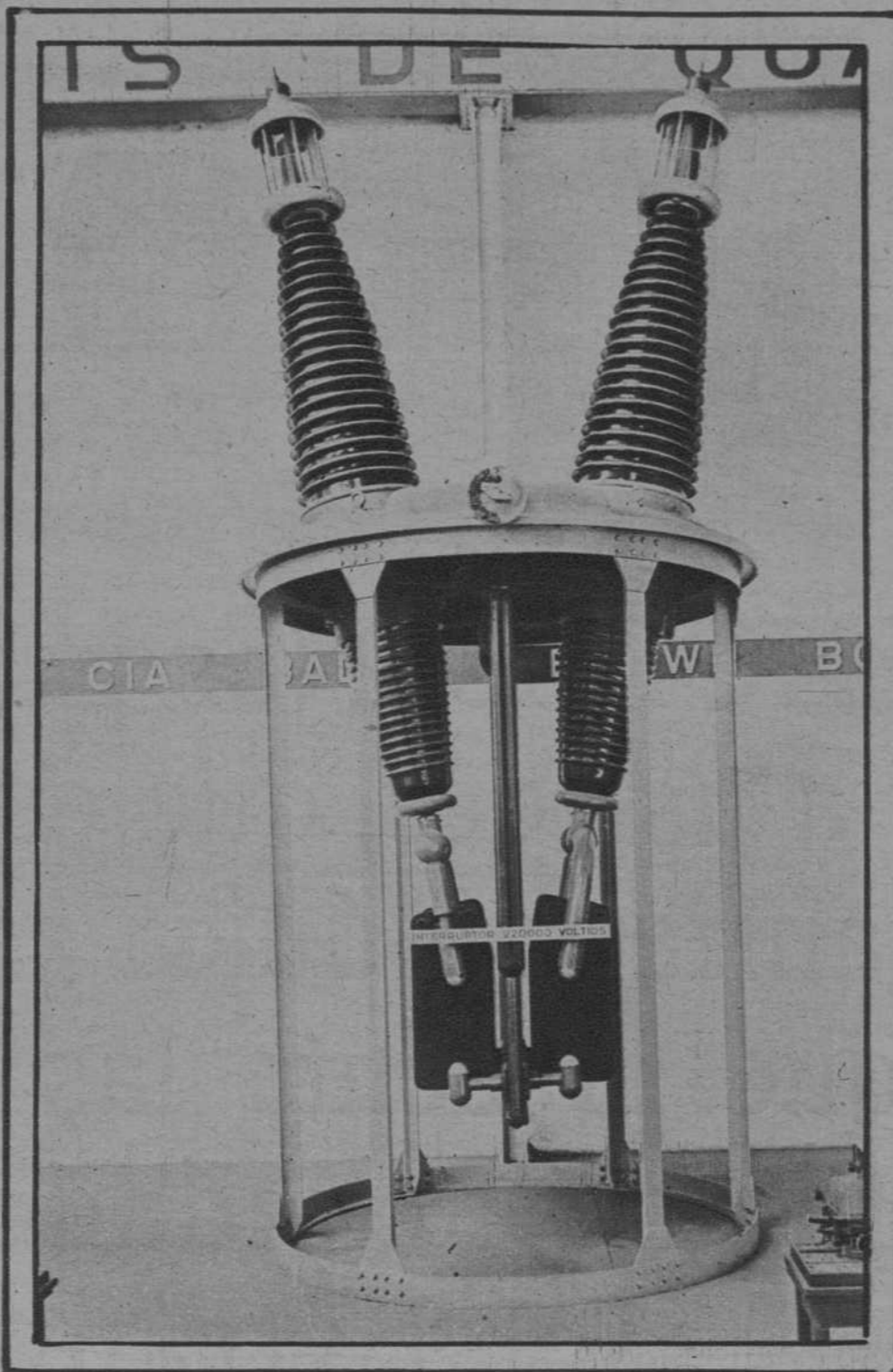
Interruptor antométrico, para 220.000 voltios. Capacidad de ruptura, 1.500.000 KVA.
