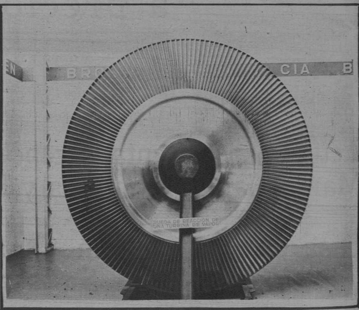
Rueda de reacción de una turbina de vapor, de 80.000 KVA.
