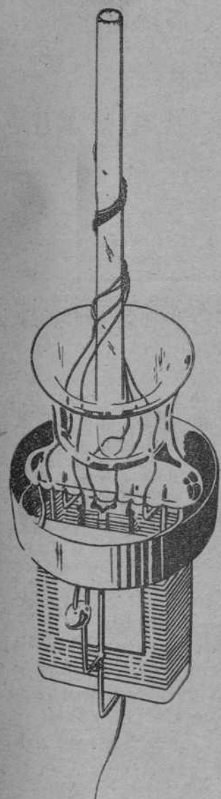
Fig. 5.—Interior de una lámpara receptora Philips a calefacción indirecta para corriente alterna tipo E 442
