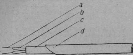
Fig. 4.—Filamento de una lámpara receptora a calefacción indirecta para corriente alterna: a - filamento, b - masa buena conductora del calor, c - tubo metálico, d - envoltura emisora de electrones
