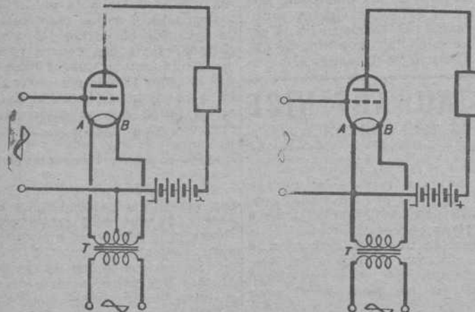
Fig. 2. Conexión incorrecta de una lámpara receptora de corriente alterna a uno de los polos de filamento.
