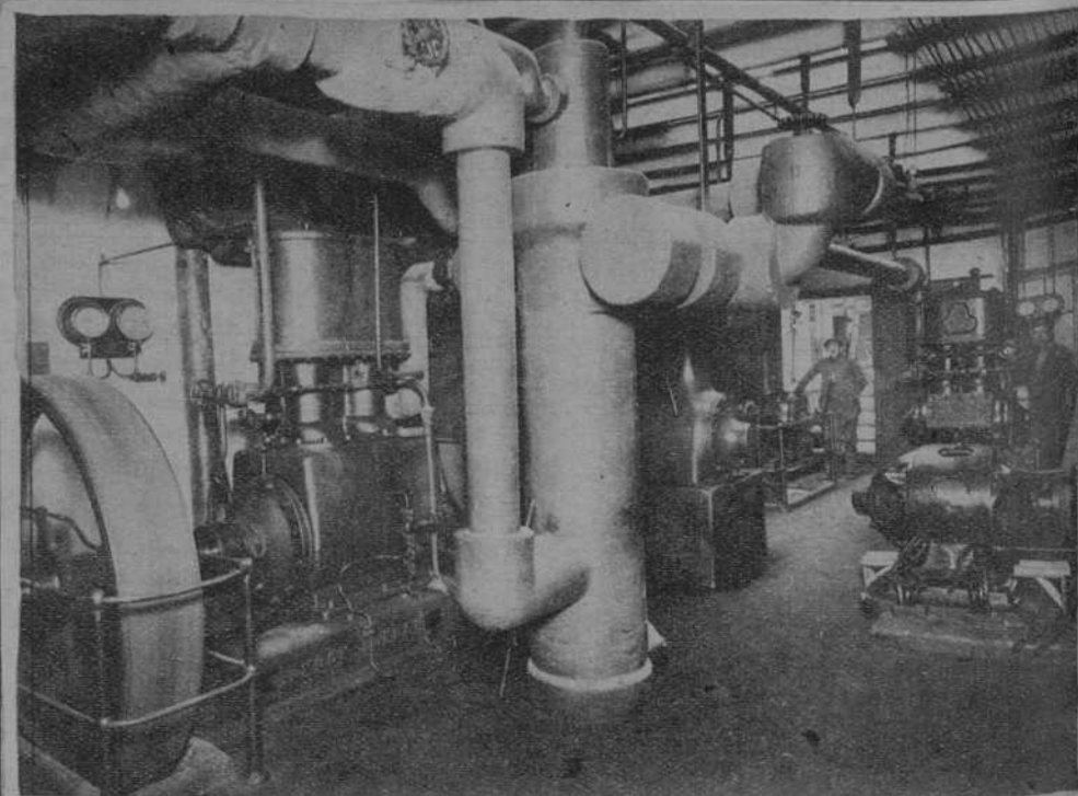
VISTAS PARCIALES DE LAS SALAS DE MAQUINAS DONDE SE PRODUCE EL FRIO
