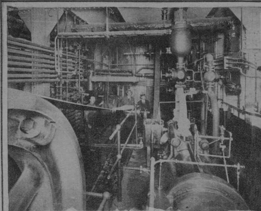
VISTAS PARCIALES DE LAS SALAS DE MAQUINAS DONDE SE PRODUCE EL FRIO
