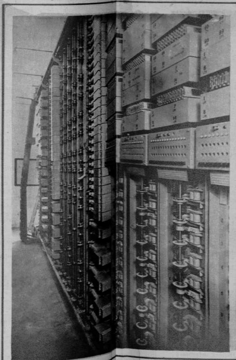
Este grupo de buscadores primeros y selectores finales completan los segundos, los inician, los primeros, la operación de enlace entre el abonado que llama y el que debe contestar.
