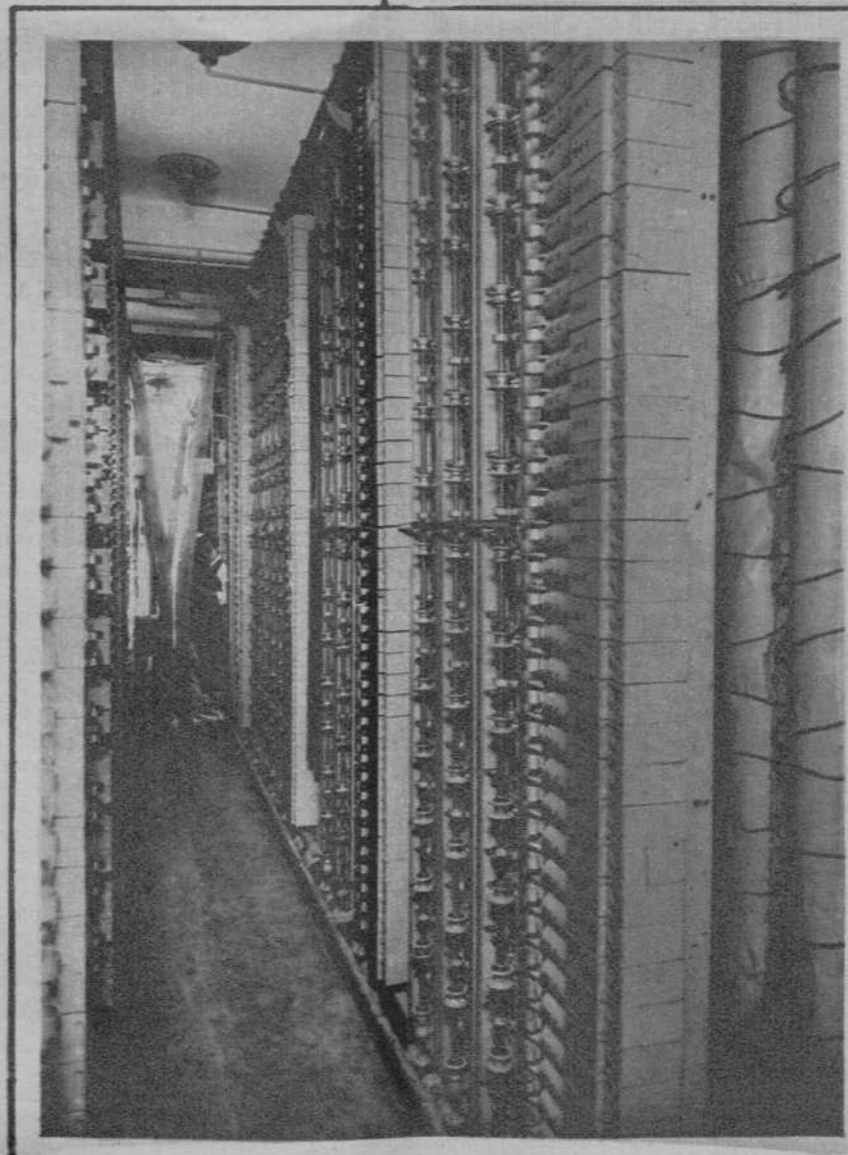
Un pasillo de selectores segundos
