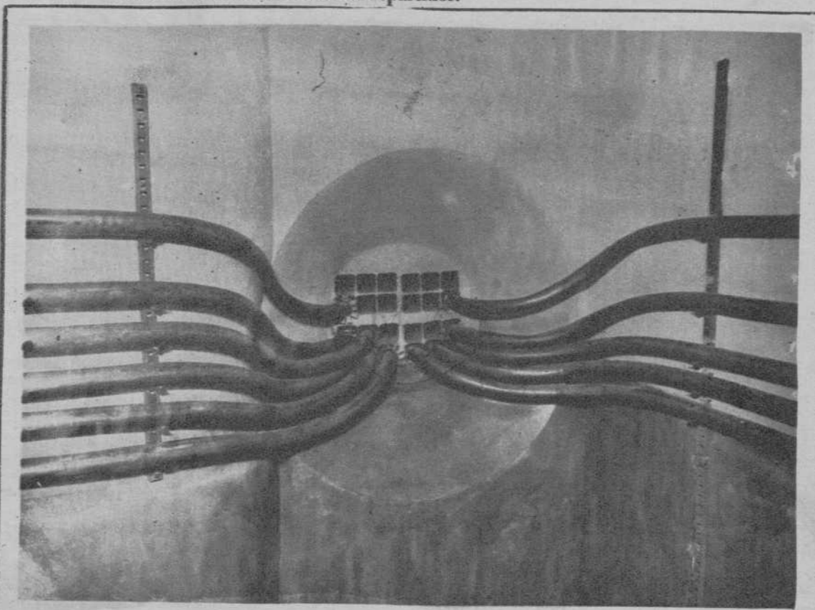
Estos once cables que entran por los once tubos ocupados de la Puerta del Angel, tienen 1.200 pares cada uno, lo que da un total de 13.000 abonados posibles para comunicar asiduamente, sin temor a cruces e interrupciones.
