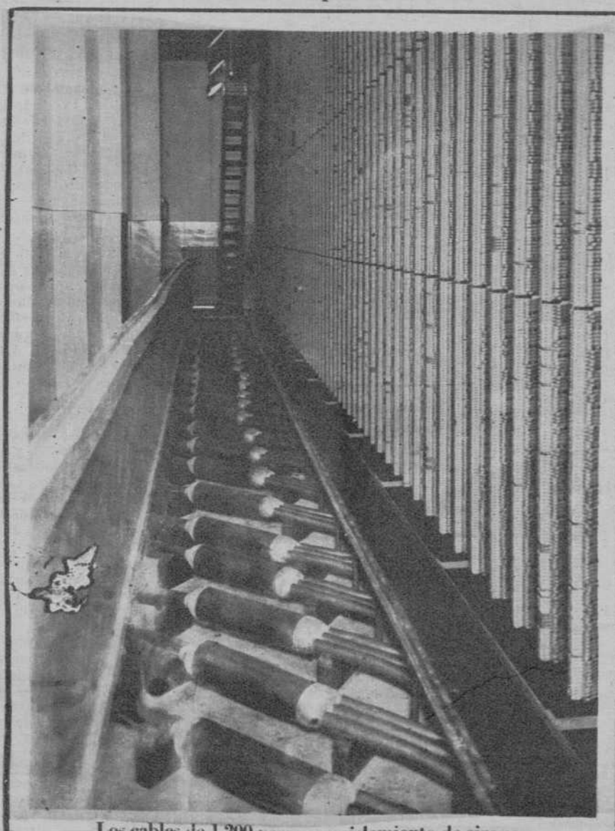
Los cables de 1.200 pares con aislamiento de aire seco llegan desde la entrada de cables a la base del repartidor, donde, en los empalmes que muestra la fotografía, se bifurcan en tres cables de 400 pares, con aislamiento de lana y seda, que terminan en las regletas verticales con protecciones.
