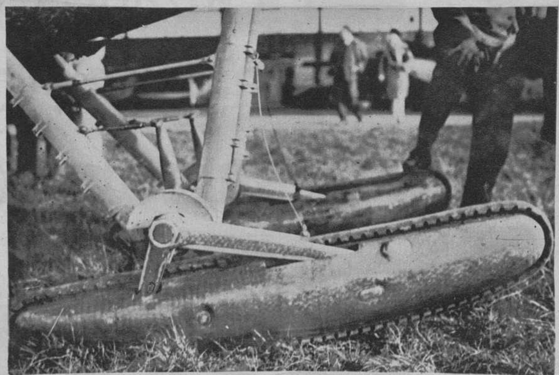
LE BOURGET (Francia).—Nuevo dispositivo para los trenes de aterrizaje de los aviones: las ruedas sustituidas por un sistema de rotación semejante al de los auto-orugas. (Fot. Consorcio).
