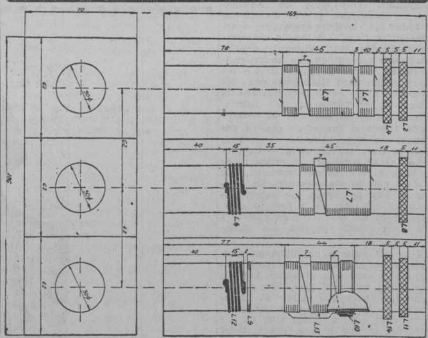
Detalles aclaratorios al esquema Tungsram, para superheterodino de seis, todas ondas, con las nuevas lámparas Tungsram 1935-36
