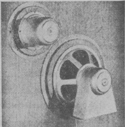
La interesantísima novedad de los Zenith: un altavoz pequeño para los agudos y otro grande para los graves, cuya sincronización produce una perfecta tonalidad. Representantes: Sánchez Ramos y Sinonetta, Pi y Margall, 5
