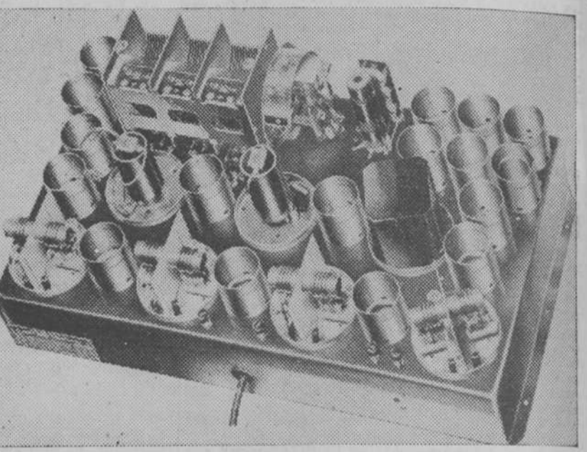
Preciosa vista del colosal Scott, que distribuye Casa Radio, de Velázquez, 31, en la que puede apreciarse la perfección y finura de su construcción
