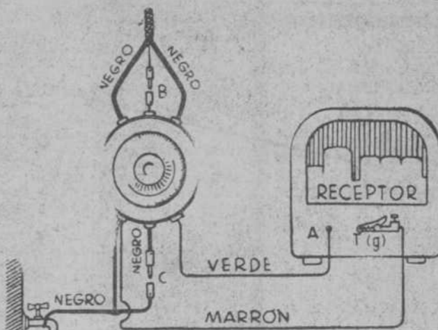
Esquema de conducción de la nueva antena antiparasitaria (patentada) Puratone Antenax, de la que nos ocupamos en otro lugar de esta sección
