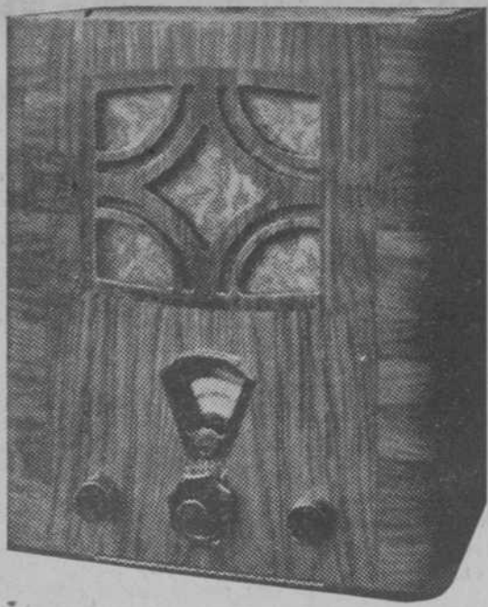
522. A.—Nuevo Super-Octodo de 6 válvulas para corriente alterna; ondas cortas y largas; equipado con la válvula octodo superada que proporciona extraordinaria selectividad y alcance; conectable a todos los voltajes; gran potencia y reproducción impecable; control antifading efectivo; regulador progresivo de tono; enchufe de "pick-up" y altavoz suplementario; moderna caja de elegantes líneas construida con maderas finas
