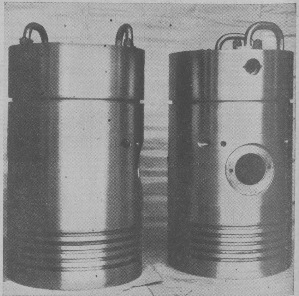
Pistones para motor Diesel de 800 HP., contruidos en Talleres Mercier, S. A., de Zaragoza
