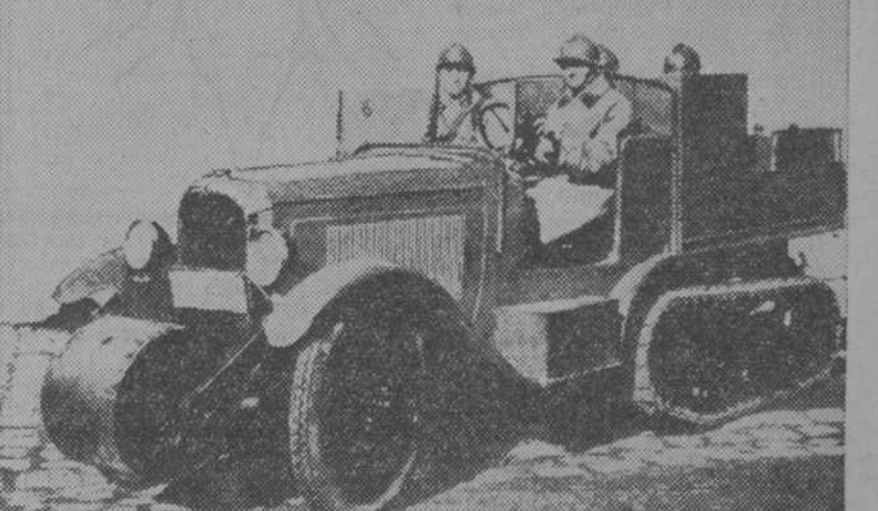
Auto-origa empleado en Francia para las unidades motorizadas
