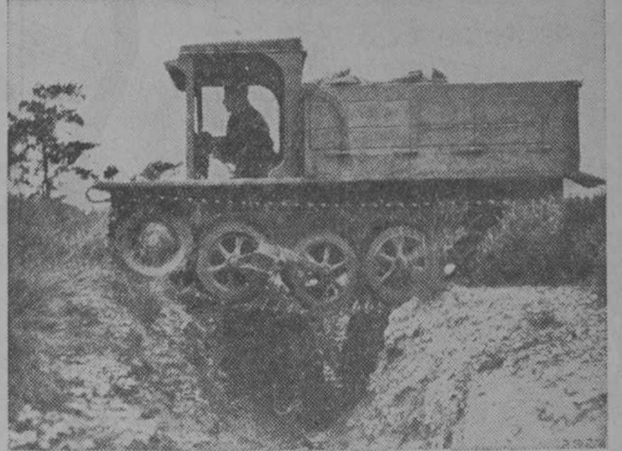
Camión "todo terreno", montado sobre un bastidor "Carden Loyd", en el momento de atravesar una torrentera
