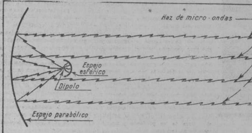
Fig. 1.—Sistema electro-óptico
