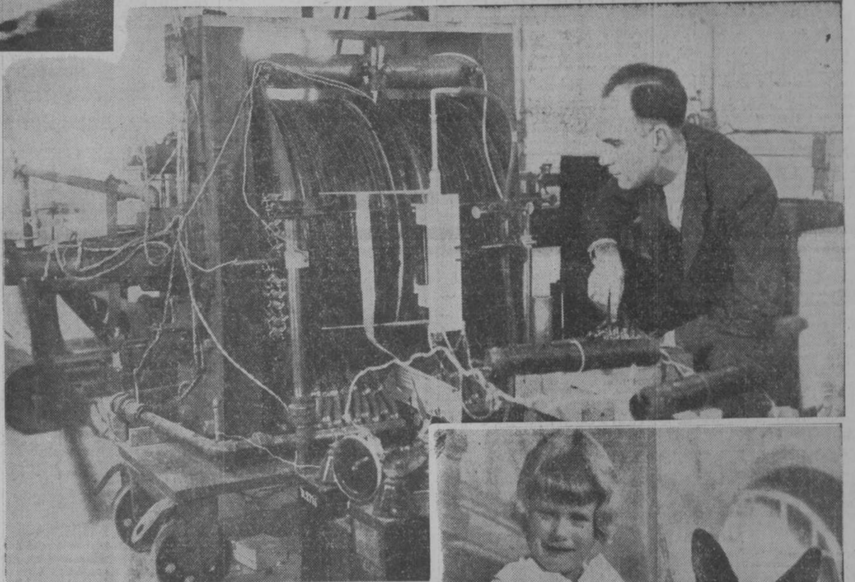
El eminente hombre de ciencia Mr. Anderson, de California, de veintiocho años, ha realizado interesante experimentos sobre la rotura del átomo mediante rayos cósmicos. En el grabado aparece en su laboratorio en el momento de fotografiar las partículas de rayos cósmicos atravesando un diafragma de plomo de once pulgadas de espesor
