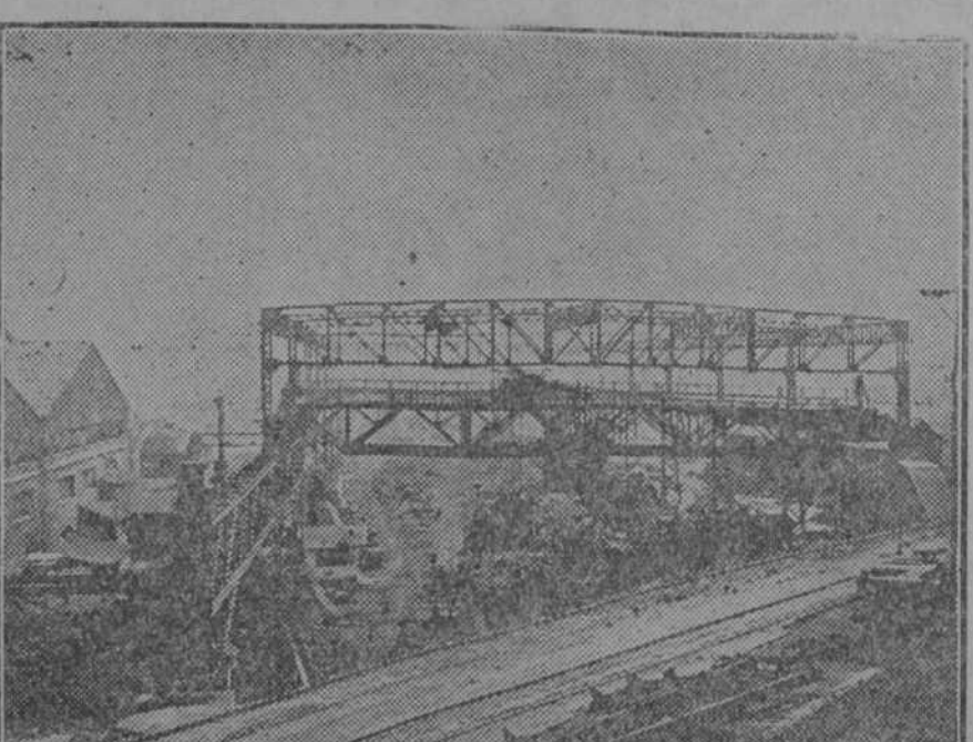
GRUA ELECTROIMAN PARA EL PARQUE DE CHATARRAS Y LINGOTES DE LA COMPAÑIA ANONIMA BASCONIA
