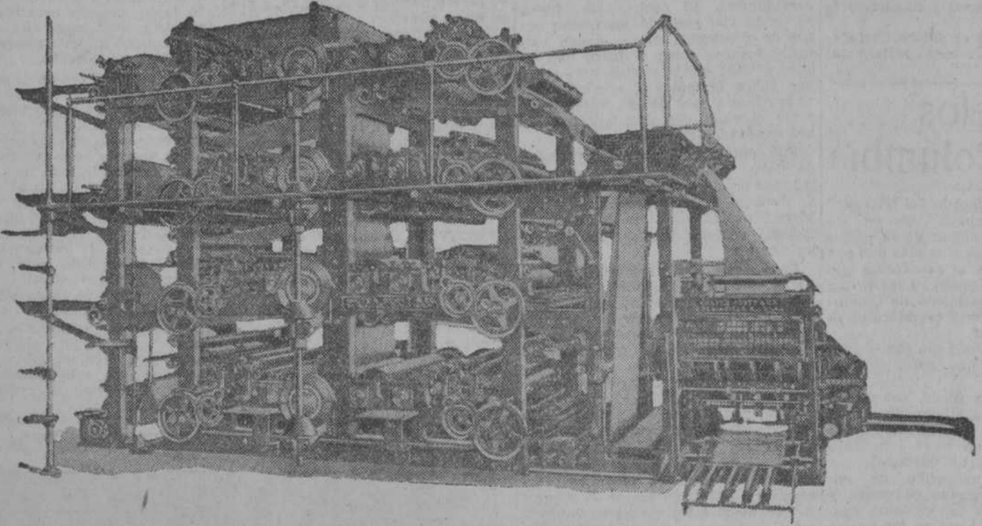
Fotograbado de la rotativa Walter Scott, con capacidad para tirar hasta 72.000 ejemplares por hora, adquirida en New-York por los propietarios de "El Siglo" y que estará en la Habana de un momento a otro. Se instalará en el edificio propiedad del Ldo. Gustavo Alonso Castañeda en construcción en la esquina de Consulado y Colón.
