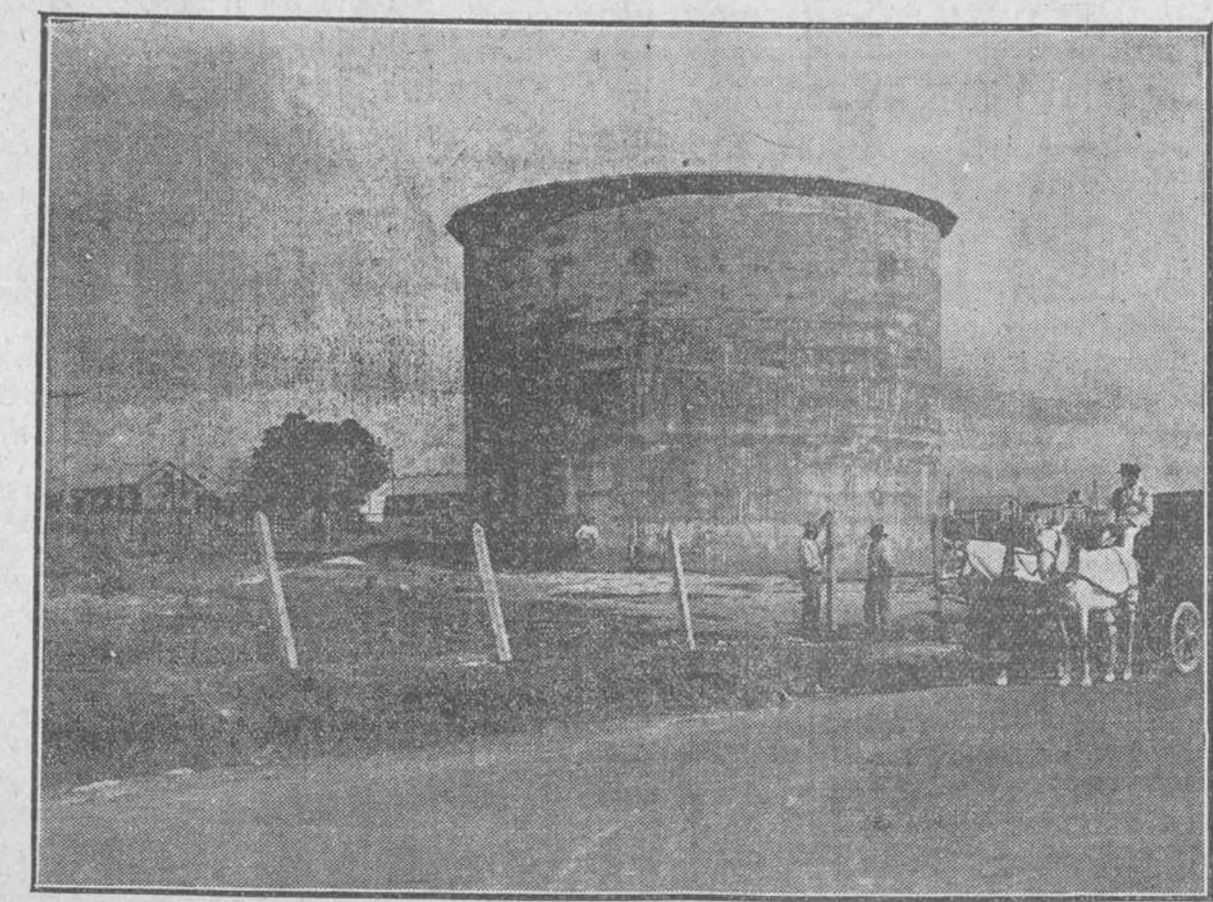
Uno de los grandes tanques del Acueducto de Marianao, cuya capacidad y sistema de filtros lo hacen una notable obra de ingeniería hidráulica, siendo su costo de $500,000.
