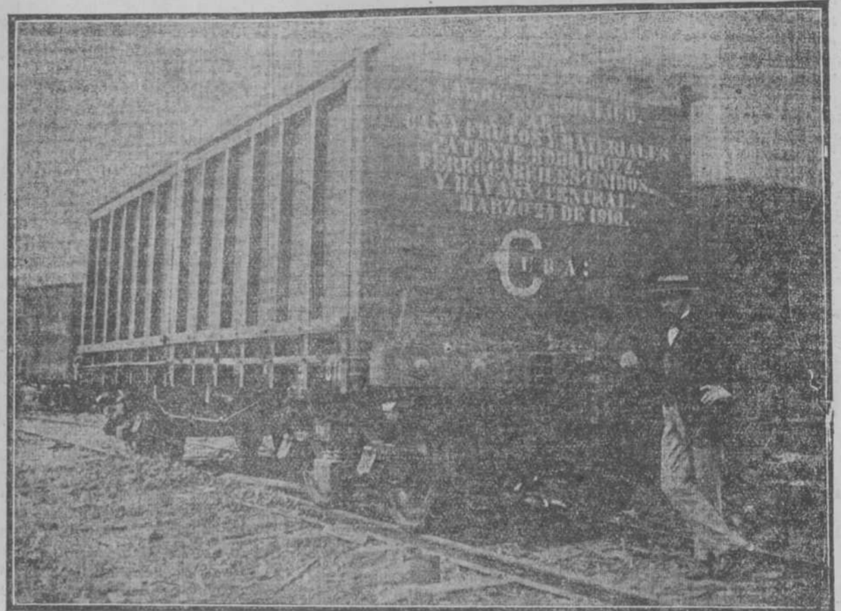
Carro automático para descargar por una banda lateral MEJORAS EN COMPUERTAS PARA CAROS.—PATENTE Ceferino Rodríguez Fernández SAN RAFAEL Y AMISTAD, APARTADO NUMERO 986.—HABANA.
