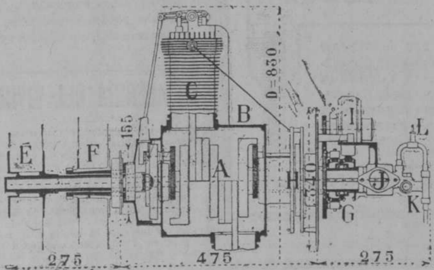
LEGENDE A, Arbre manivelle; B, Carter; C, Cylindre; D, Distribution; EF, Hélices; G, Commande de la magneto; H, Distributeur d'allumage; I, Magneto; J, Bride du carburateur; K, Pompe a huile; L, Pulseur.
