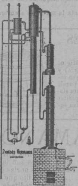
Aparato destilación continua á fuego directo. Producción del alcohol de 95 á 96°, 6 sean 40° Cartier.
