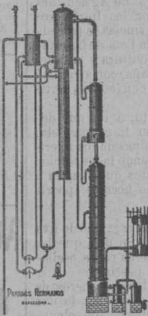
Aparato destilación continua á vapor. Producción del alcohol de 95 á 96°, 6 sean 40° Cartier.
