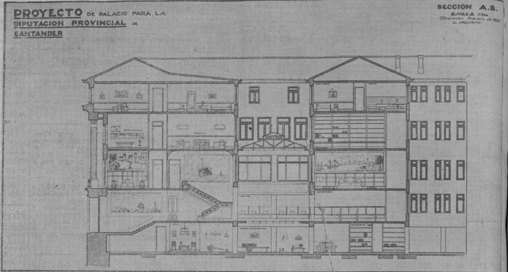
Sección del Palacio de la Diputación provincial, proyecto del notable arquitecto señor Bringas.
