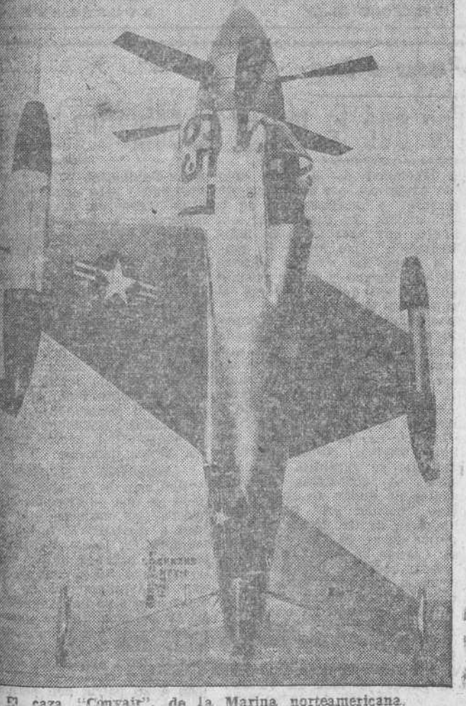
El caza "Convair", de la Marina norteamericana.
