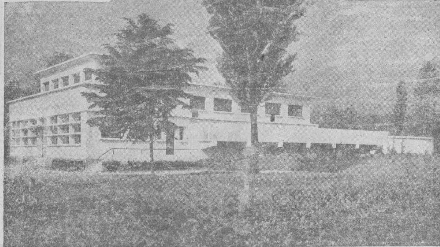
He aquí una vista general de la Estación Clarificadora de Viry-Chatillon, para el abastecimiento de aguas de París. De la que será una reproducción la que se va a construir en Salamanca.—Arriba, a la izquierda, galería de gobierno de mandos de la Estación; a la derecha, el accetator, instalación la más moderna para la clarificación.
