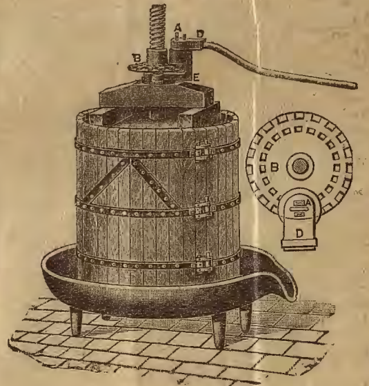
PRENSA PARA VINO de especial construcción de AVERLY, S. A.
