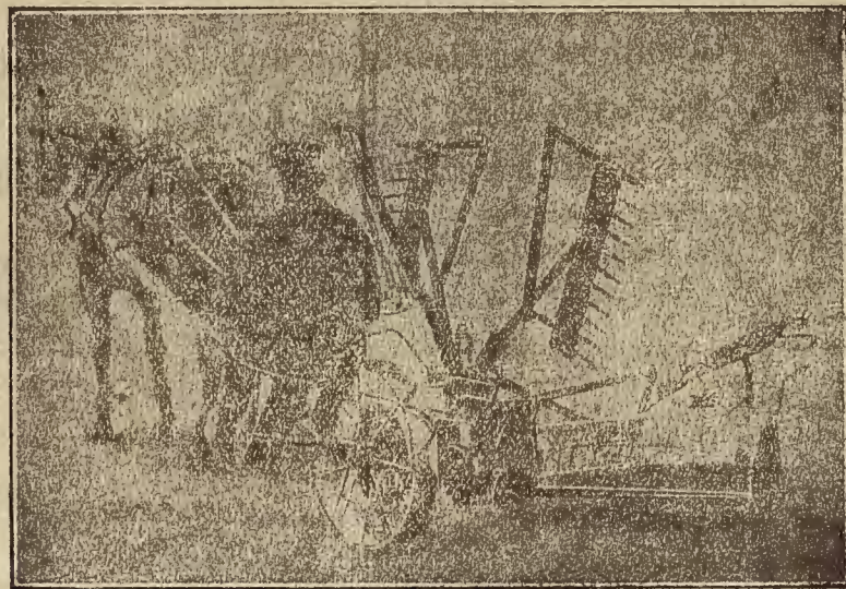
Agavilladora de una mula La Golondrina. Única que trabaja en terrenos quebrados y entre arbolado.
