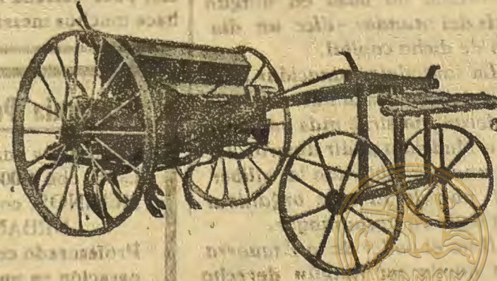
Sembradora-abonadora con avantren, marca LABAD
