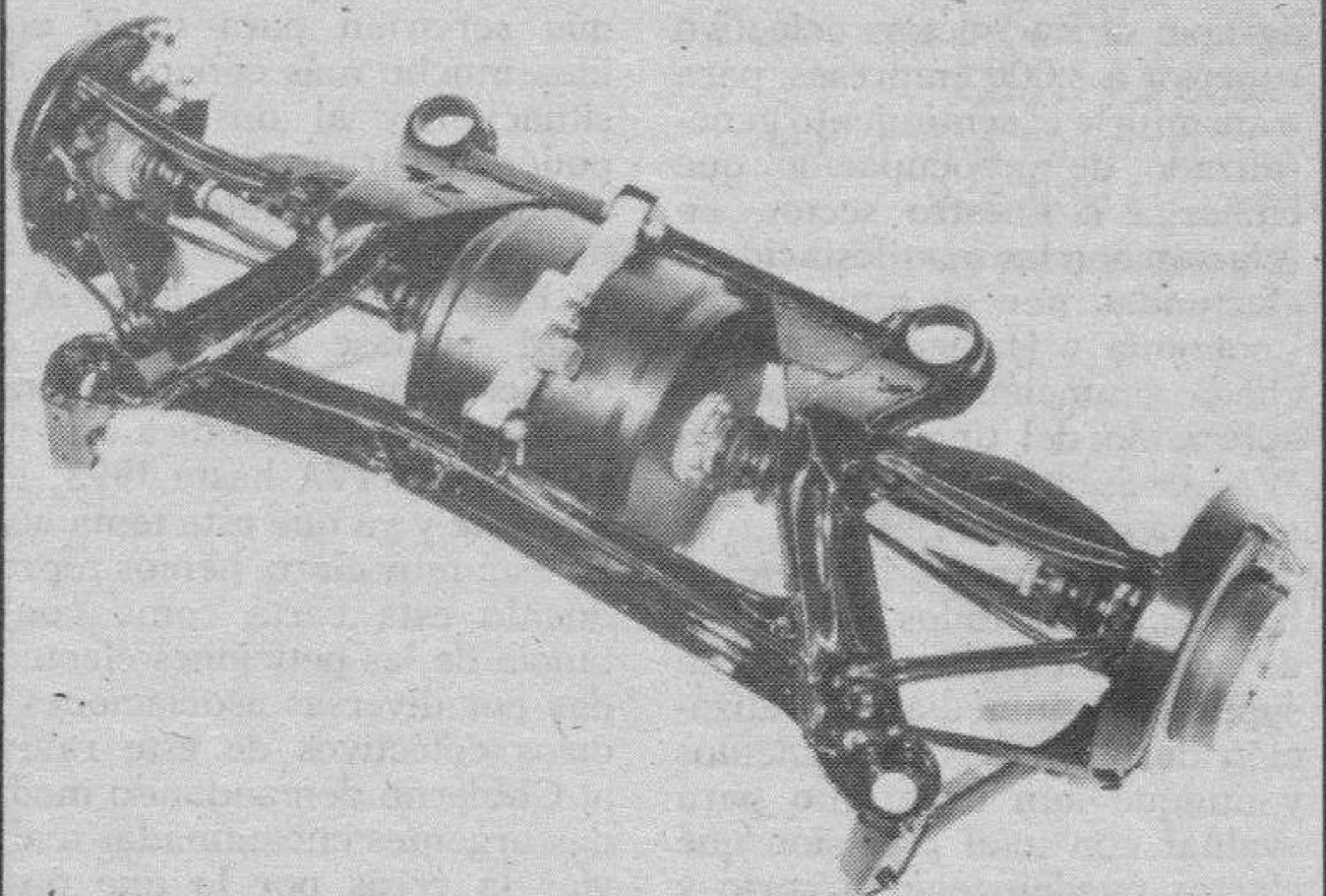
Este sistema adecuado especialmente para uso en ciudad, prescinde de muchos elementos del motor de combustión. (Foto: DB).
