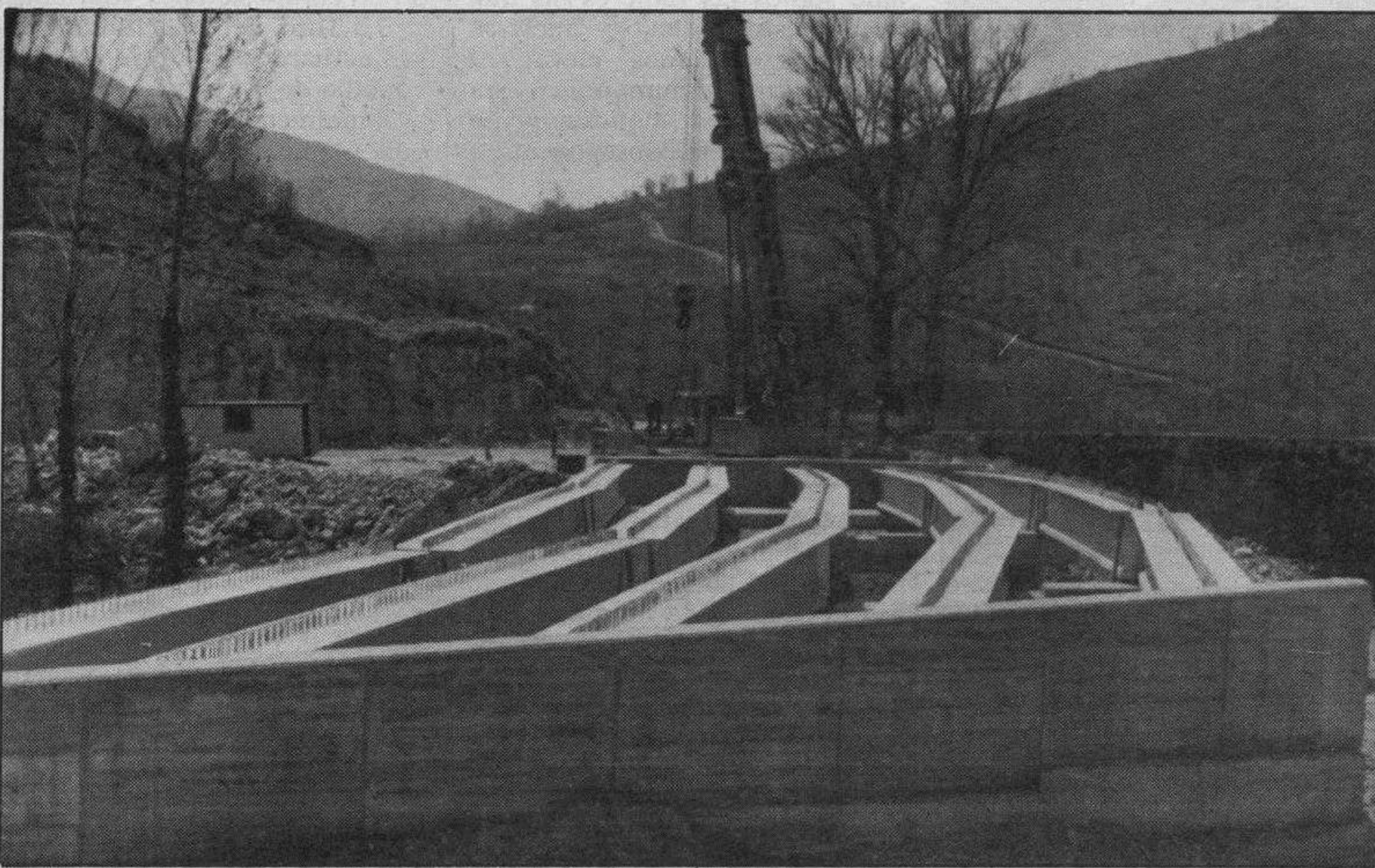
Vigas del puente nuevo sobre el Rudrón. (Foto: J.C.P.)
