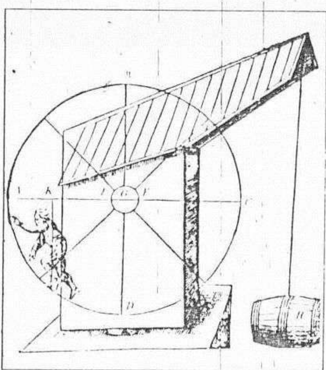
Artificio para pesar un tonel, de Simon Stevin (1548-1620). El peso del hombre equilibra el del barril, cuatro veces mayor.
