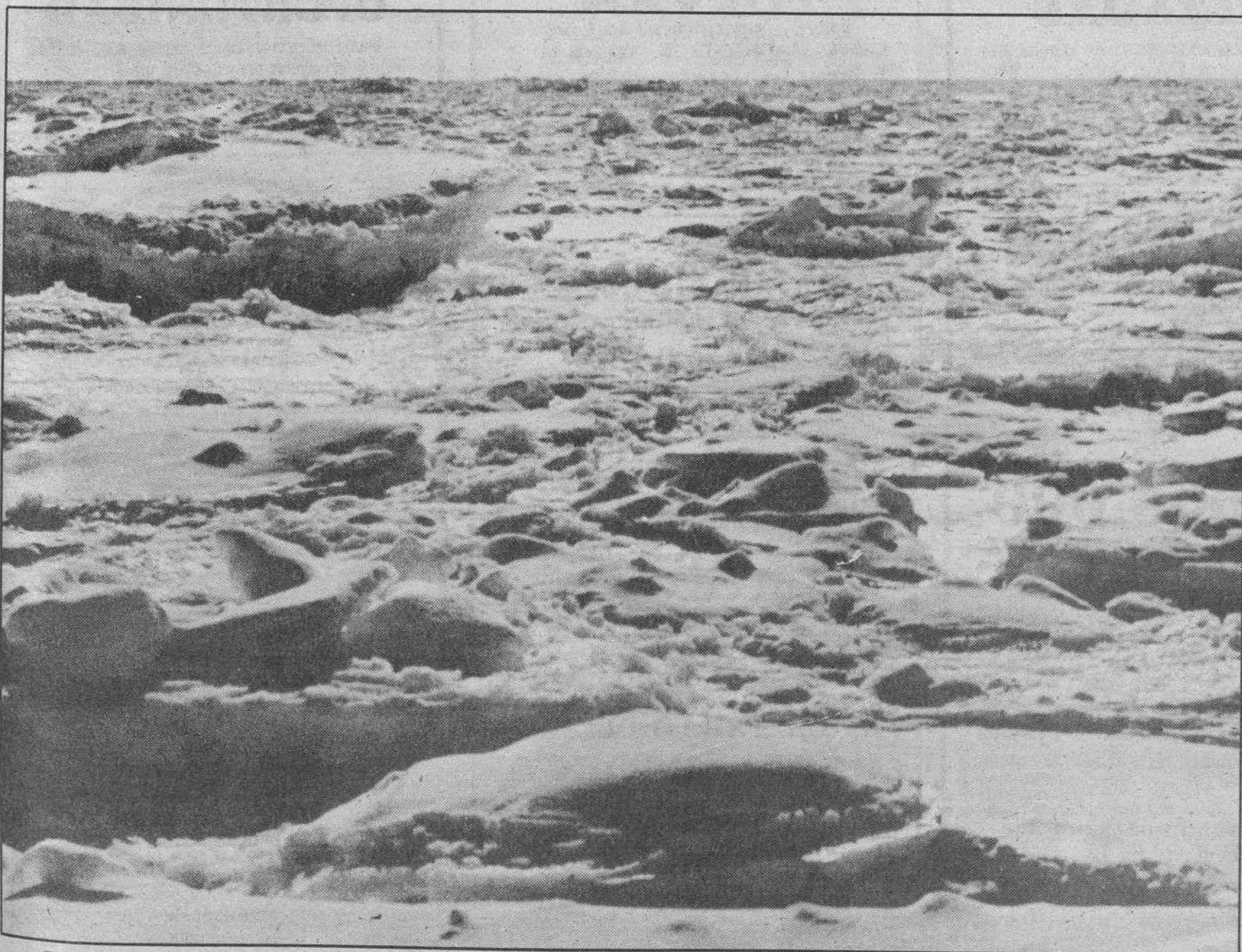
Es posible que el dióxido de carbono y el metano aumenten la temperatura de la Tierra y que comience un deshielo en amplias zonas. Foto Archivo
