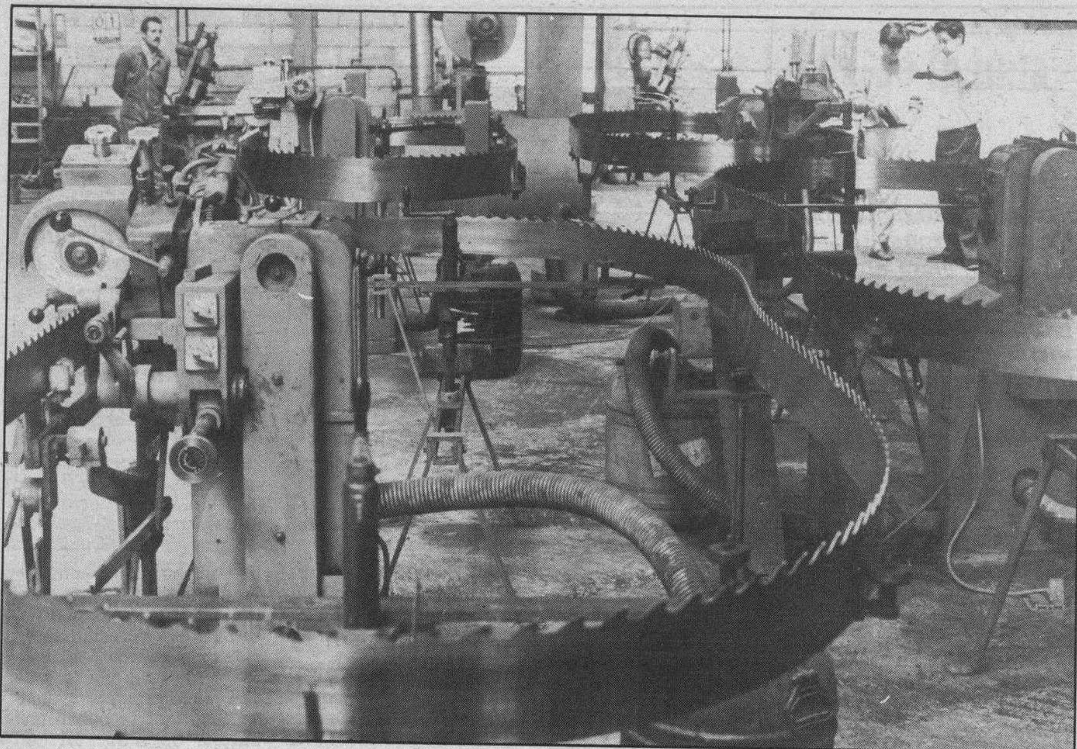
CAR, S.A. durante el proceso de reafilado de varias sierras de cinta.
