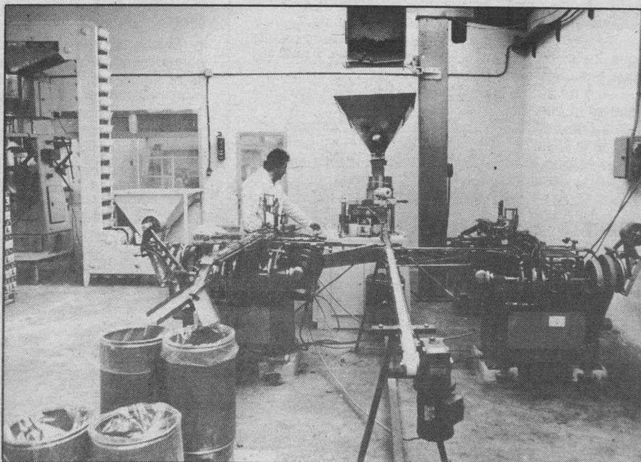
Máquina mezcladora.
