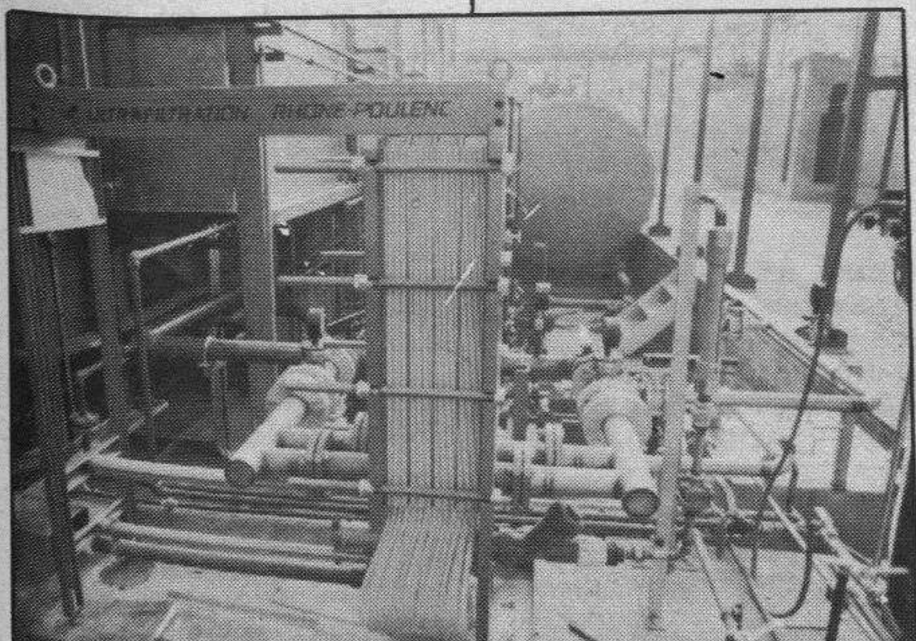
Detalle del ultrafiltro.
