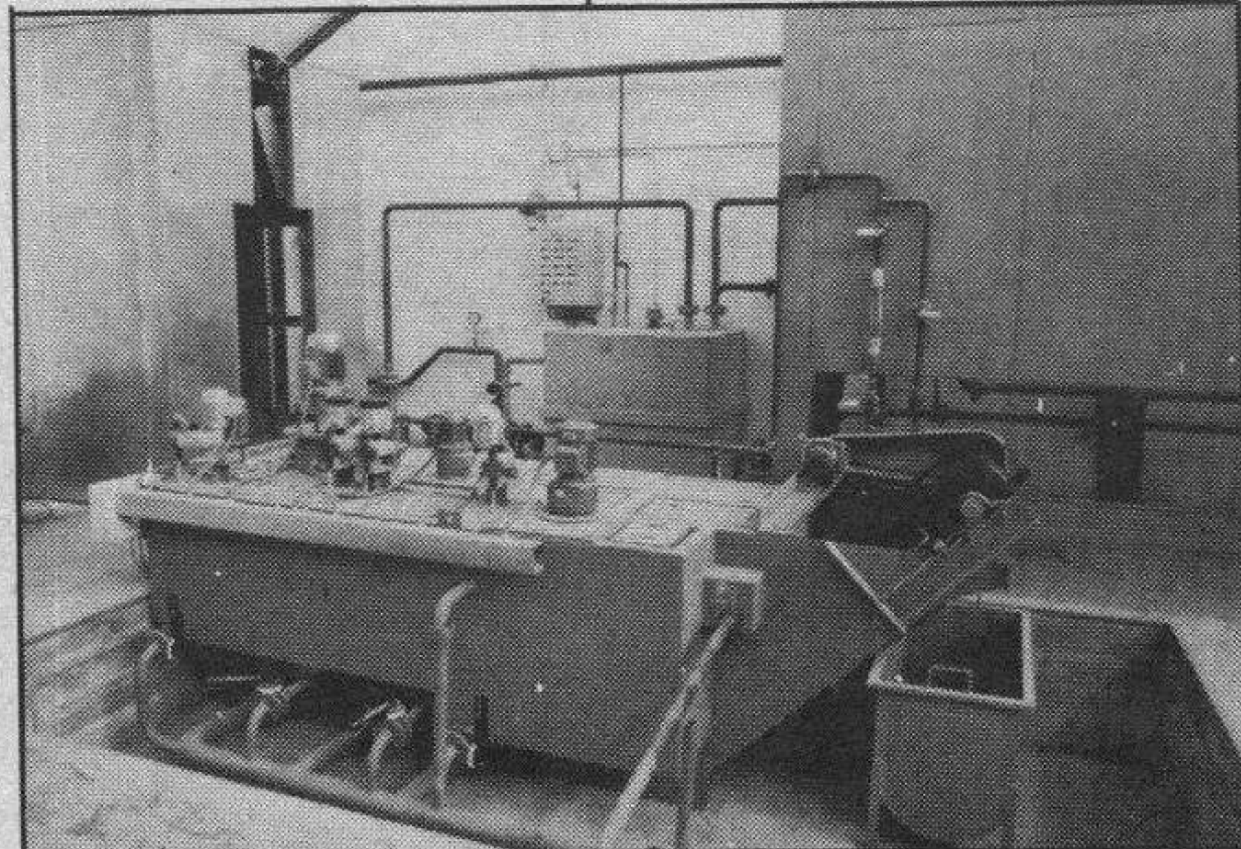
Instalación de tratamientos de vertidos líquidos.
